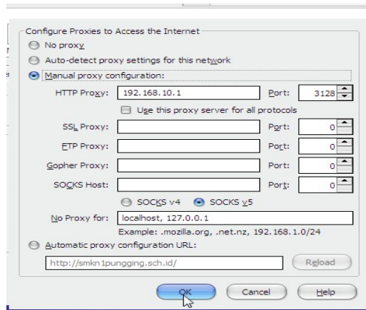
Gambar 11.1 Tampilan Konfigurasi
